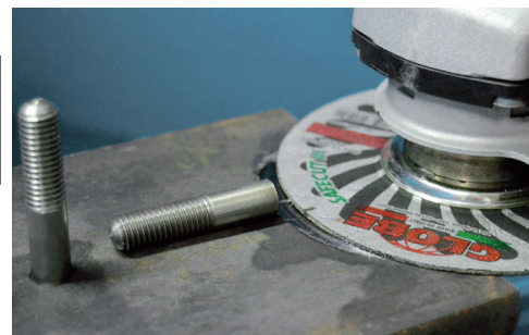
Taglio raso di prigionieri. Flush cutting of stud bolts.
