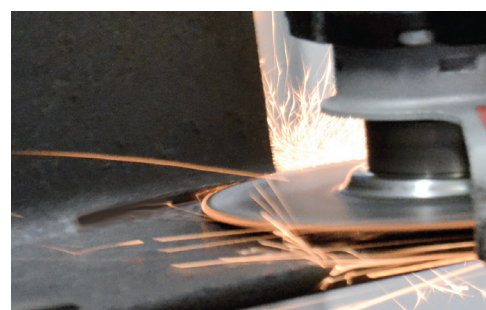
Taglio raso di profilo ad "H" in acciaio. Flush cutting of H-shaped steel sections.
